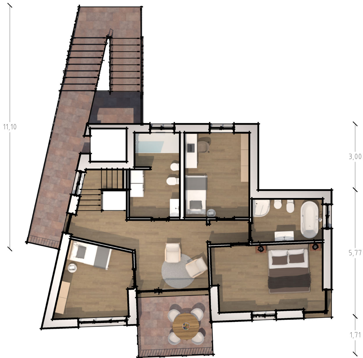
PIANO SECONDO sc. 1:100
