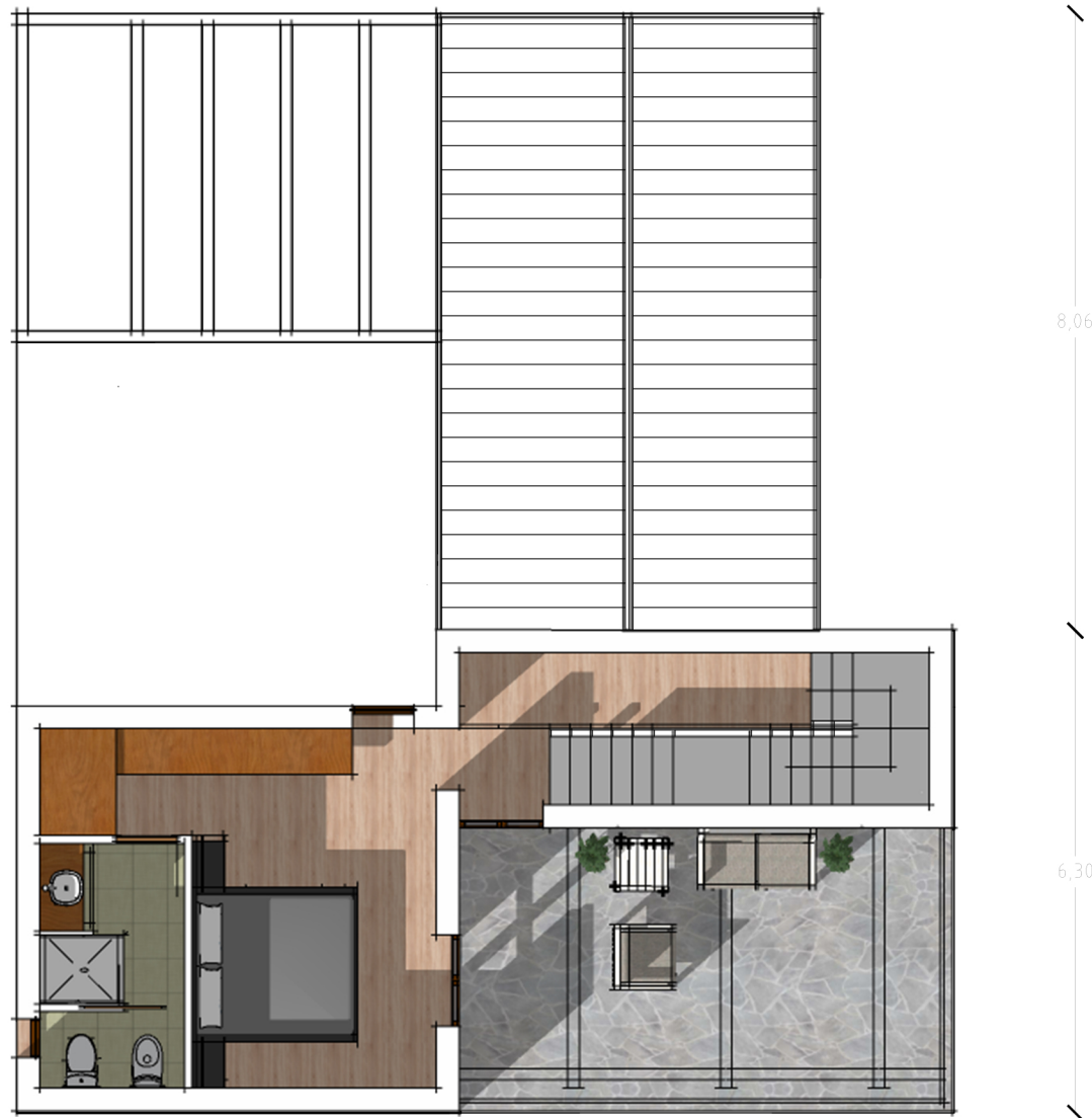
PIANO PRIMO sc. 1:100
