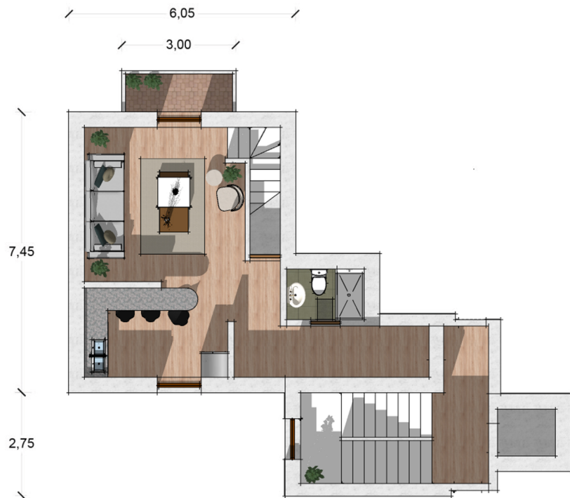
PIANO PRIMO sc. 1:100
