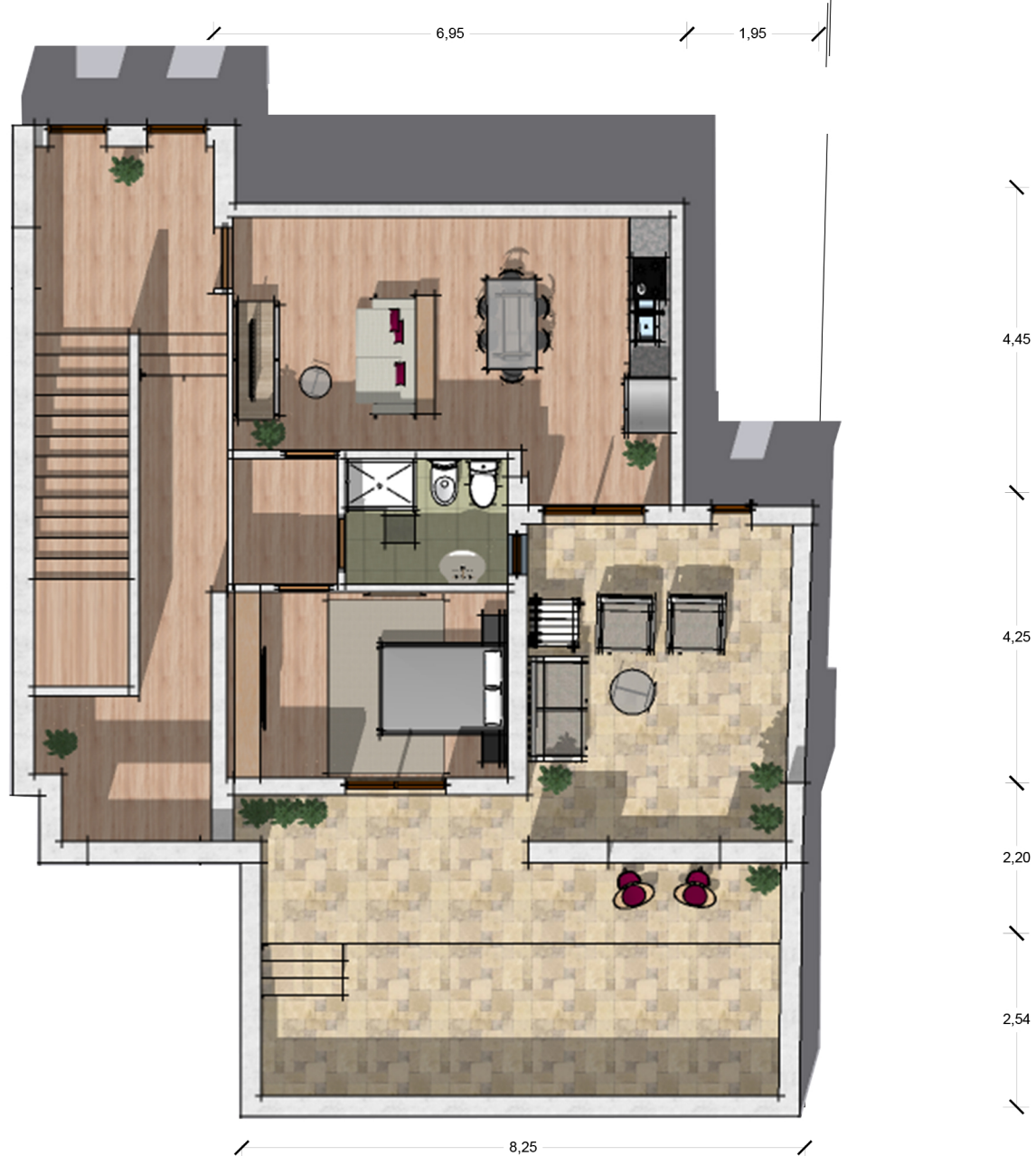
PIANO TERRA sc. 1:100
